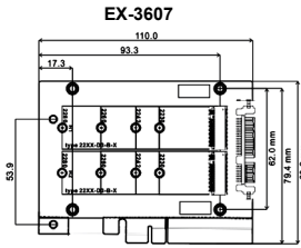
M.2 NFGG Modul B-Key
